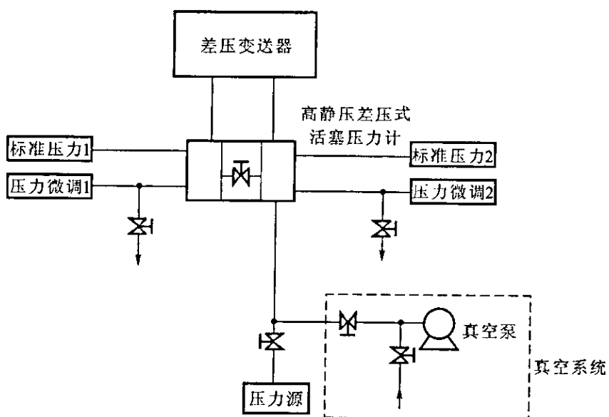
图 A-5 差压变送器输入部分的连接
