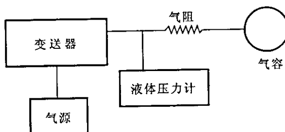
图 A-3 气动压力变送器输出部分的连接
